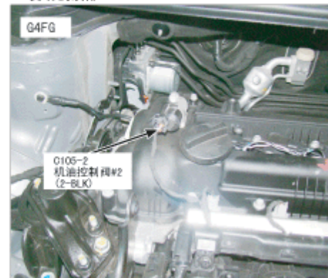
18. 发动机顶部
